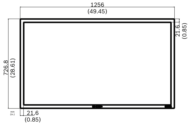
UML-423-90: Frontansicht
