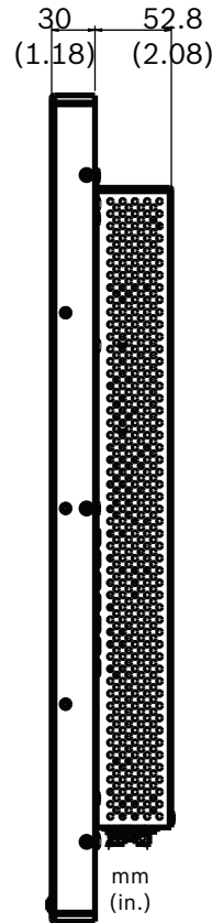
UML-423-90/UML-553-90: Seitenansicht
