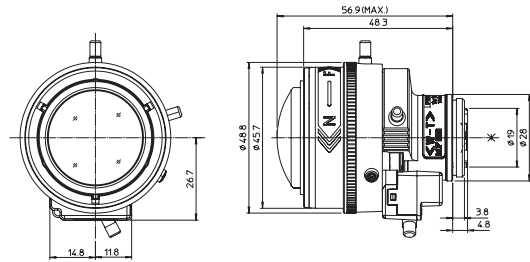
Unit : mm
