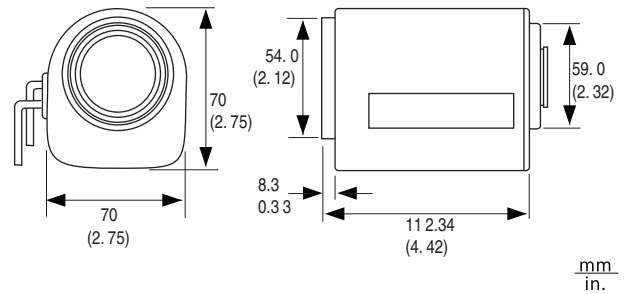
Abmessungen LTC 3384/21
