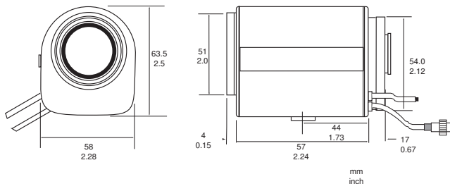
Abmessungen LTC 3283/20
