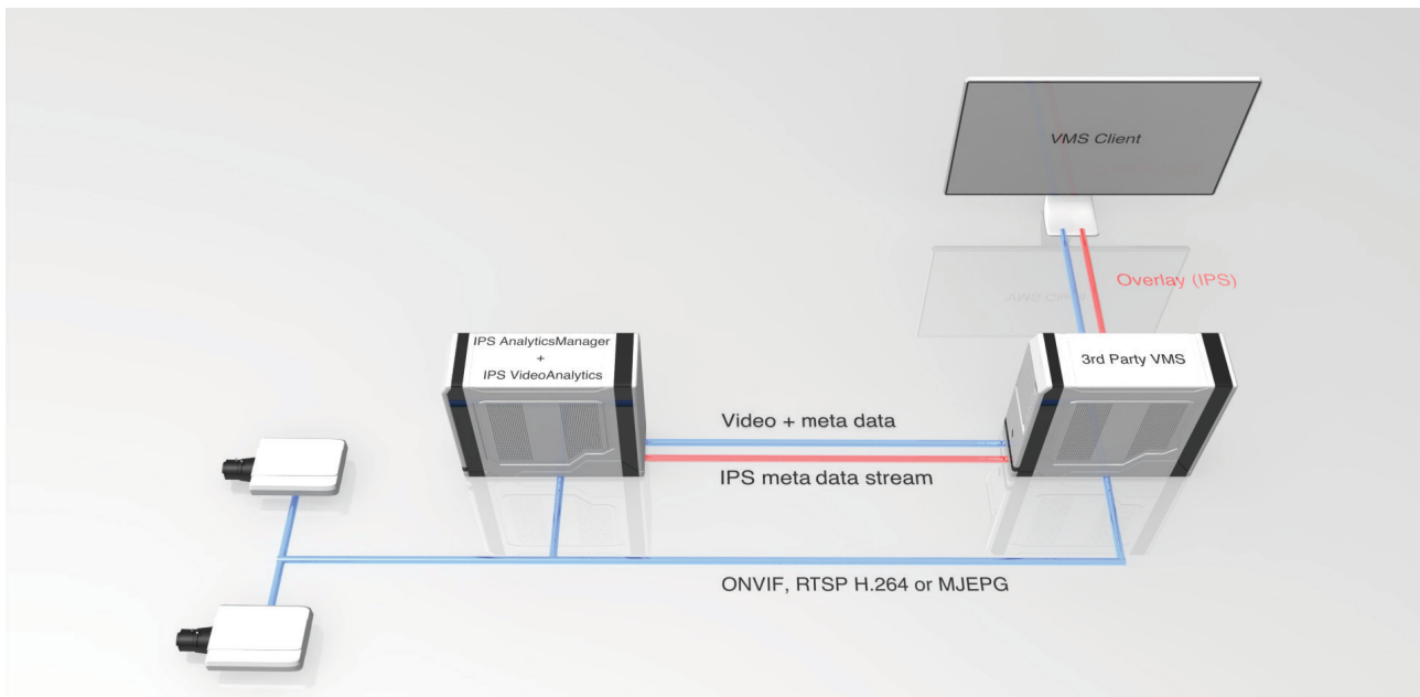
Oben: Mögliche Variante der Integration von IPS VideoAnalytics in Videomanagementsysteme von Drittanbietern mittels IPS AnalyticsManager (Server.)
